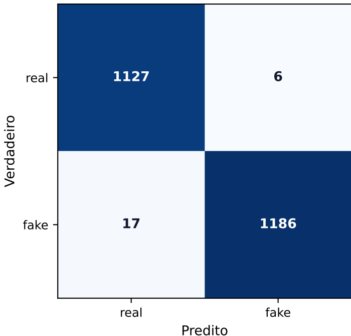
Matriz de confusão — MultiscaleCNN
