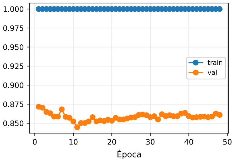
Acurácia
