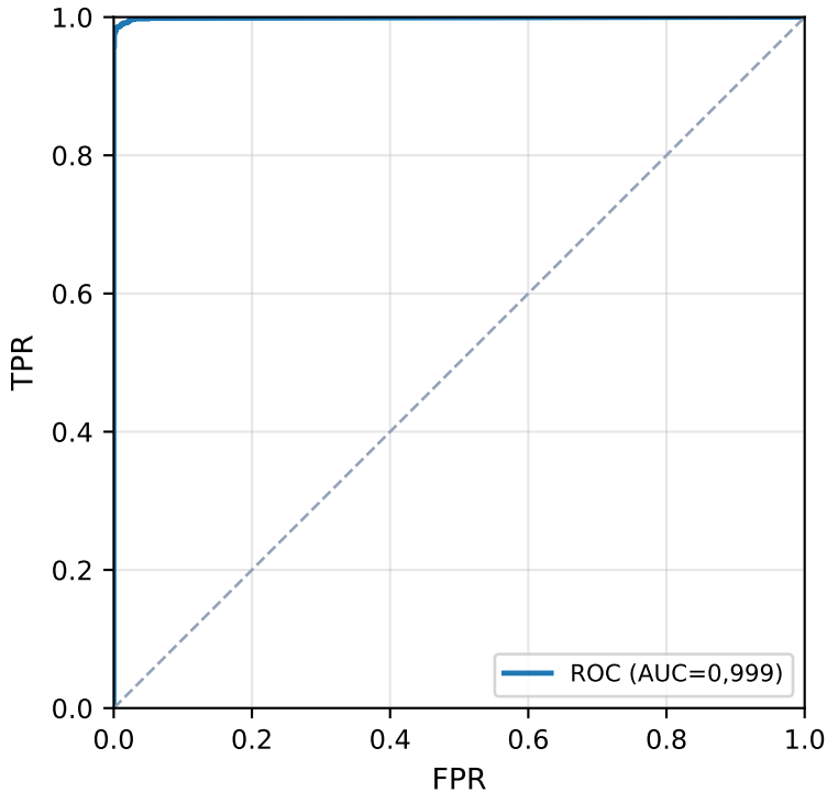
ROC — MultiscaleCNN
