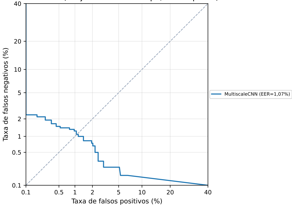
Curvas DET (conjunto de teste limpo, escala probit)
