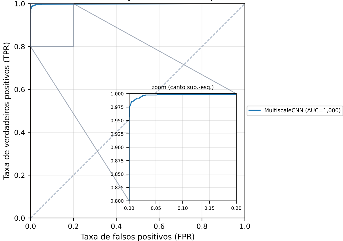
Curvas ROC (conjunto de teste limpo)
