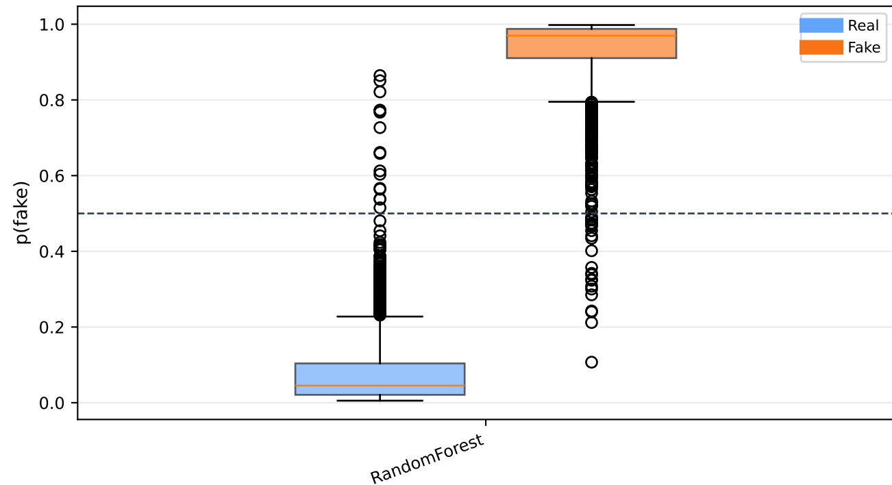
Distribuição dos scores por classe real
