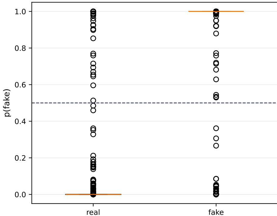
Scores por classe — RawNet2
