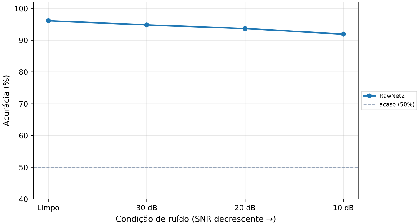
Robustez sob ruído AWGN
