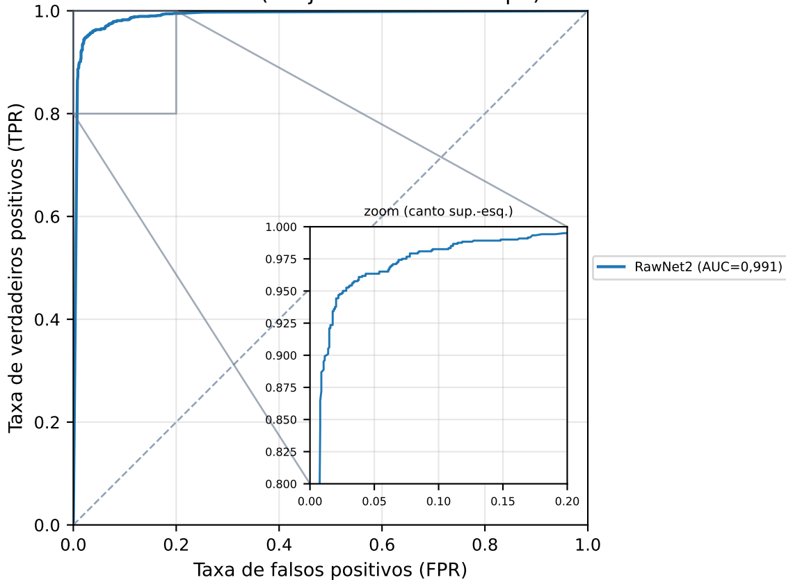
Curvas ROC (conjunto de teste limpo)
