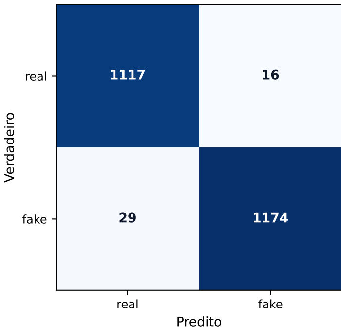
Matriz de confusão — SVM
