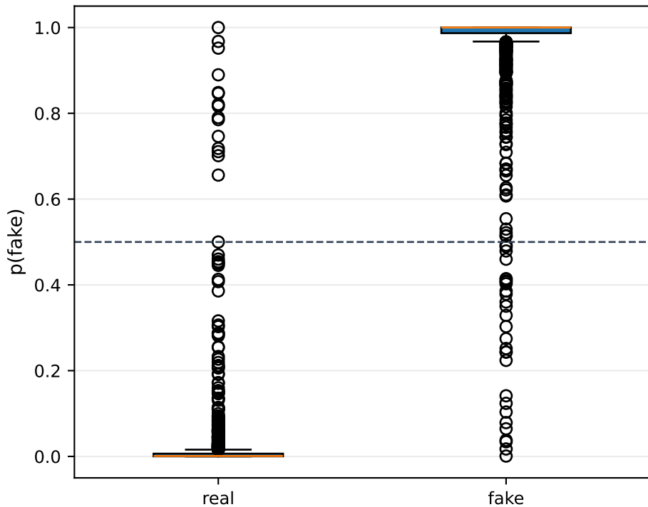
Scores por classe — SVM
