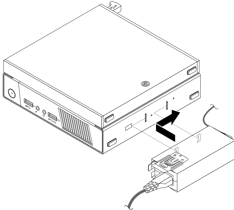
Figure 16. Installation du système de retenue du boîtier d'alimentation
