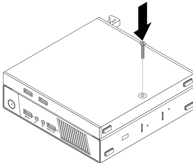
Figure 37. Installation de la vis de fixation du boîtier d'E-S
