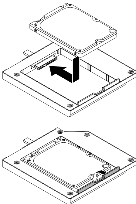
Figure 30. Installation d'une nouvelle unité de disque dur dans le système de retenue
