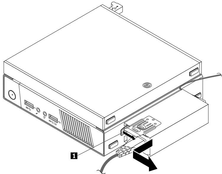
Figure 15. Retrait du système de retenue du bloc d'alimentation
