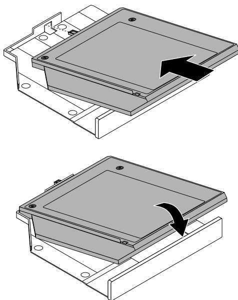
Figure 31. Installation de la carte de l'unité de disque dur dans le système de retenue
