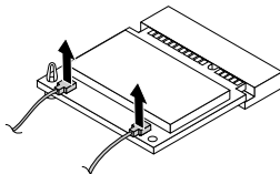
Figure 49. Retrait des câbles du module de carte Wi-Fi
