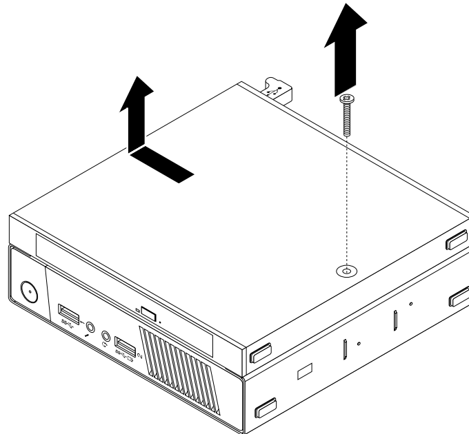
Figure 25. Retrait du coffret du disque optique
