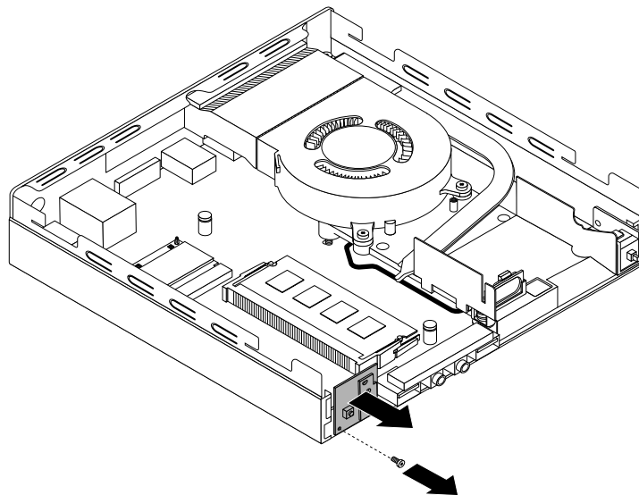
Figure 47. Retrait de la carte du bouton d'alimentation
