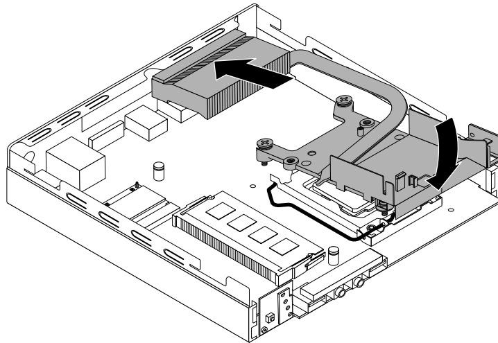
Figure 69. Positionnement du nouveau module thermique
