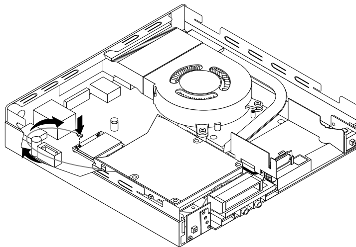
Figure 56. Installation du câble de l'antenne Wi-Fi avant
