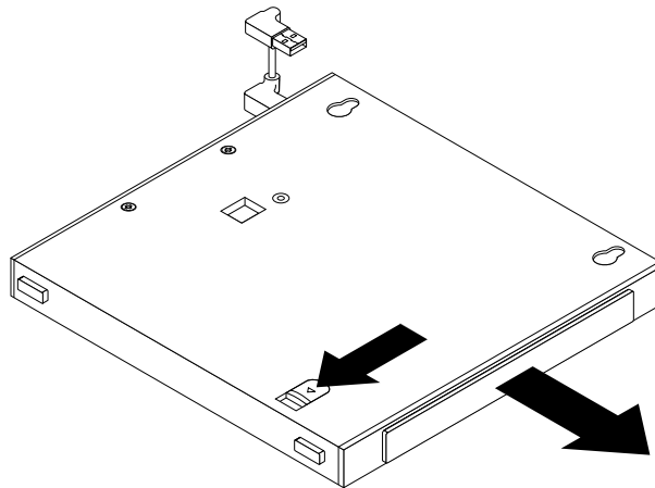
Figure 26. Retrait de la carte de l'unité de disque dur secondaire dans le coffret du disque optique
