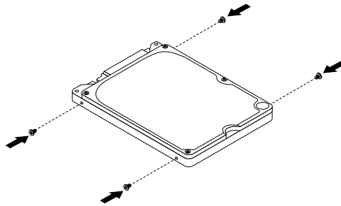
Figure 29. Installation des vis sur l'unité de disque dur
