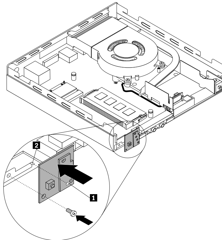
Figure 48. Installation de la carte du bouton d'alimentation
