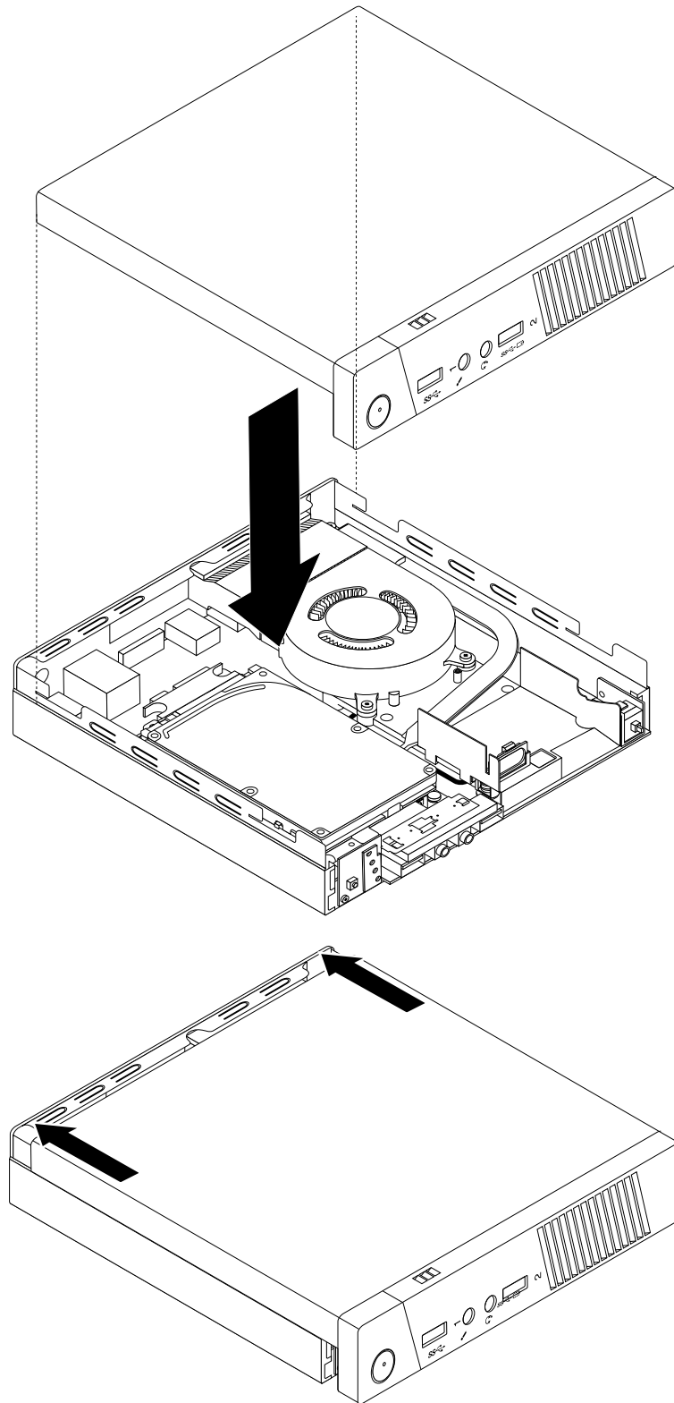
Figure 74. Installation du carter de l'ordinateur
