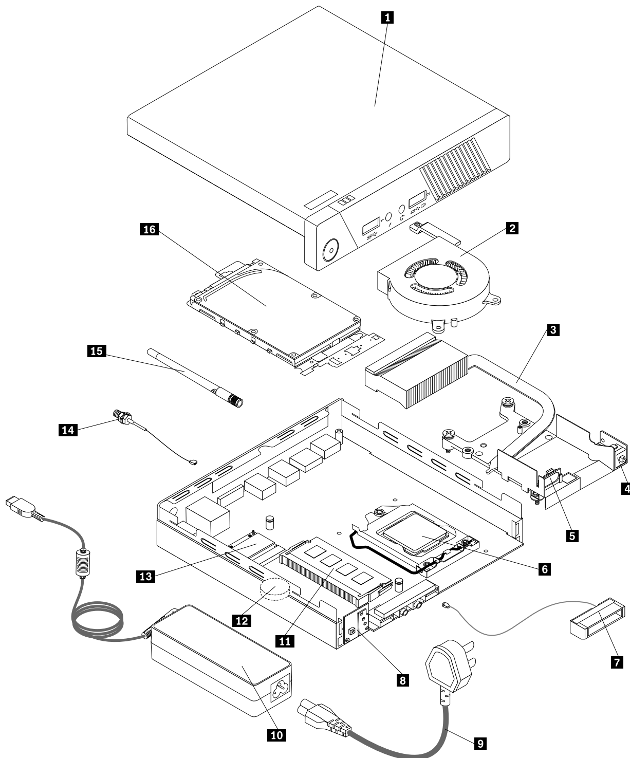
Figure 3. Emplacement des composants
