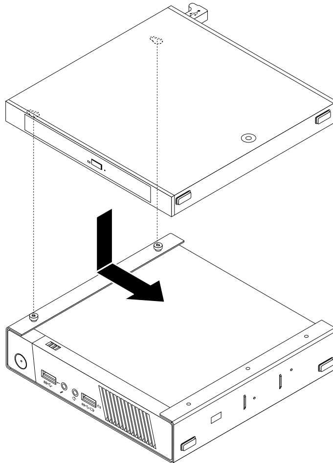
Figure 23. Installation du coffret du disque optique
