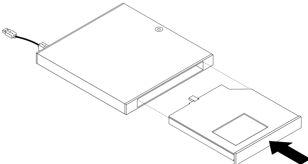
Figure 32. Installation du système de retenue dans le coffret du disque optique
