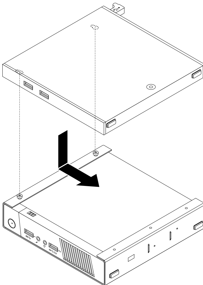
Figure 36. Installation du boîtier d'E-S
