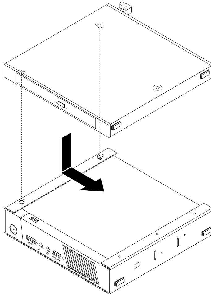
Figure 33. Installation du coffret du disque optique
