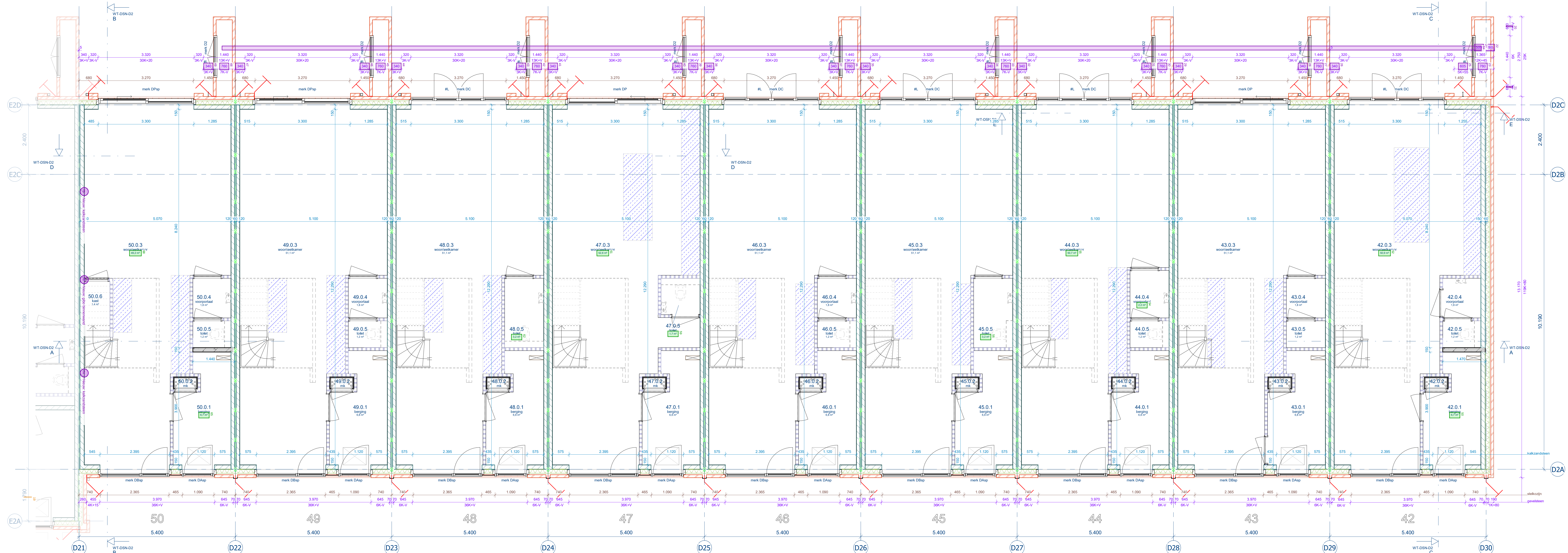
begane grond schaal 1 : 50
