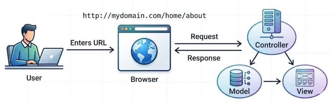
Hình 2: Minh họa luồng yêu cầu của người dùng trong ASP.NET MVC
