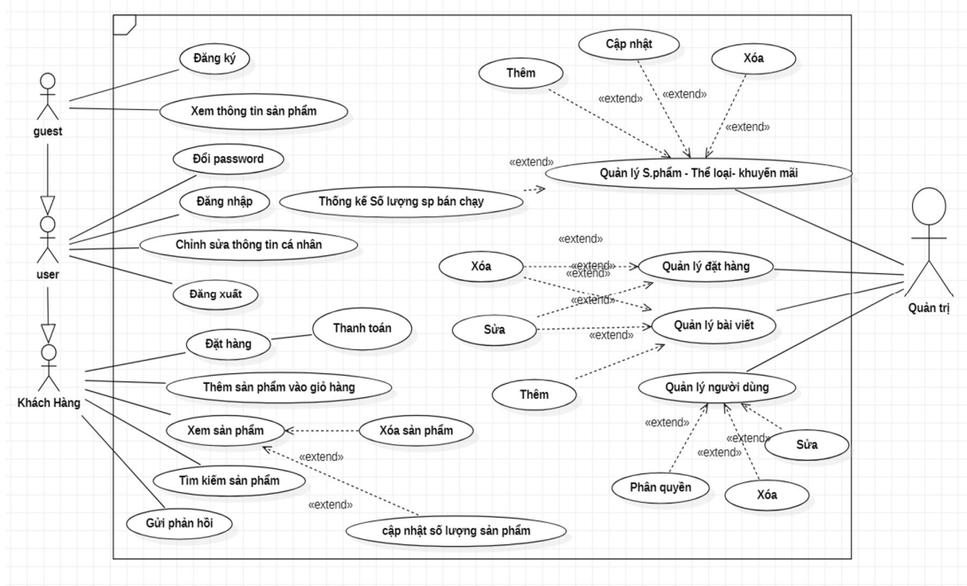
Hình 5: Biểu đồ Use – Case mức độ tổng quát
