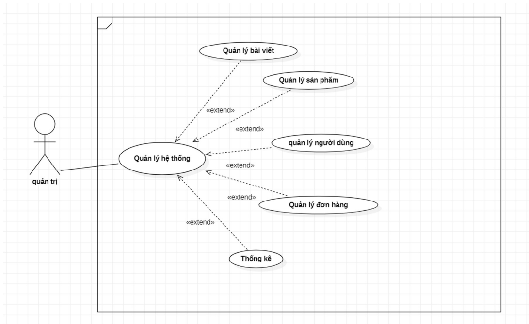
Hình 6: Biểu đồ Use – Case quản lý hệ thống
