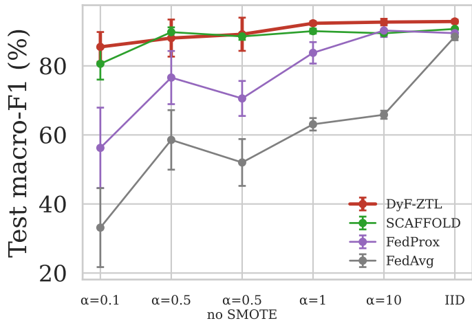
(b) Macro-F1
