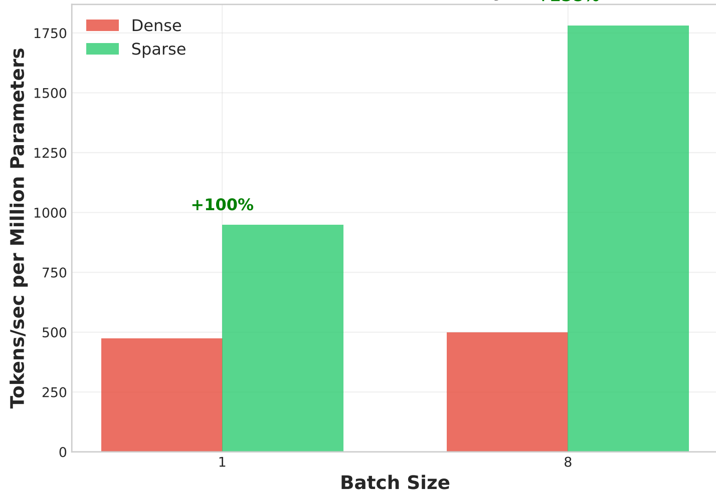
Parameter Efficiency +258%
