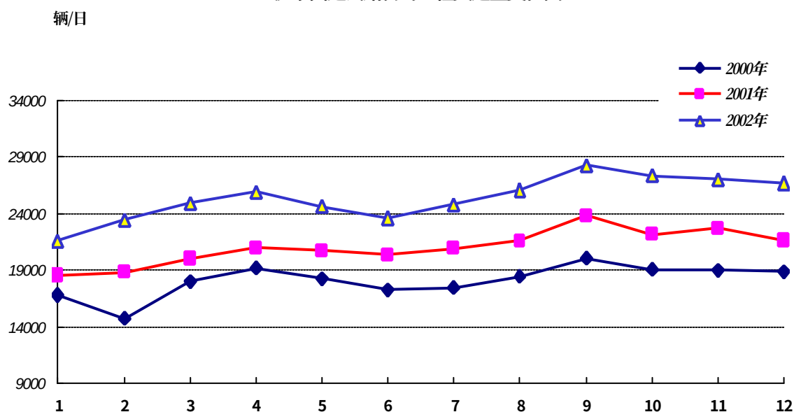
沪宁高速公路日均全程交通量变化图
