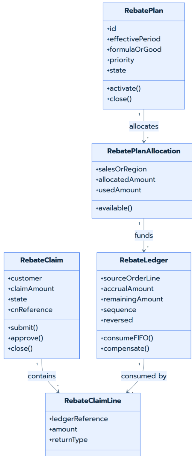
ภาพที่ 4 – Rebate domain UML
