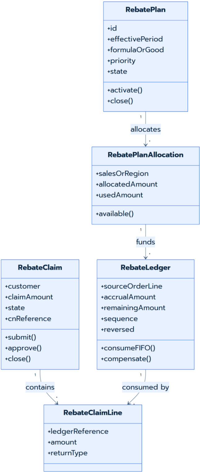
ภาพที่ 4 – Rebate domain UML
