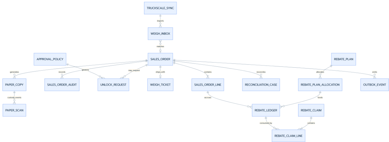
ภาพที่ 2 – Operational ERD and evidence relationships
