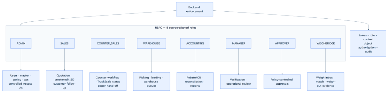
ภาพที่ 3 – Source-aligned RBAC responsibility map
