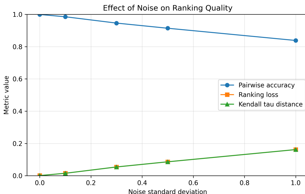
Hình 4: Ảnh hưởng của độ lệch chuẩn nhiễu đến chất lượng ranking. Khi nhiễu tăng, pairwise accuracy giảm, trong khi ranking loss và Kendall tau distance tăng.
