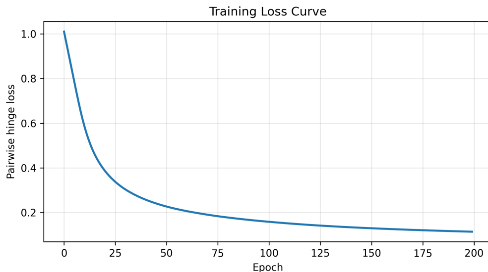
Hình 2: Đường cong pairwise hinge loss trong quá trình huấn luyện. Loss giảm nhanh ở các epoch đầu và tiếp tục giảm chậm dần về sau, cho thấy quá trình tối ưu đang hội tụ.
