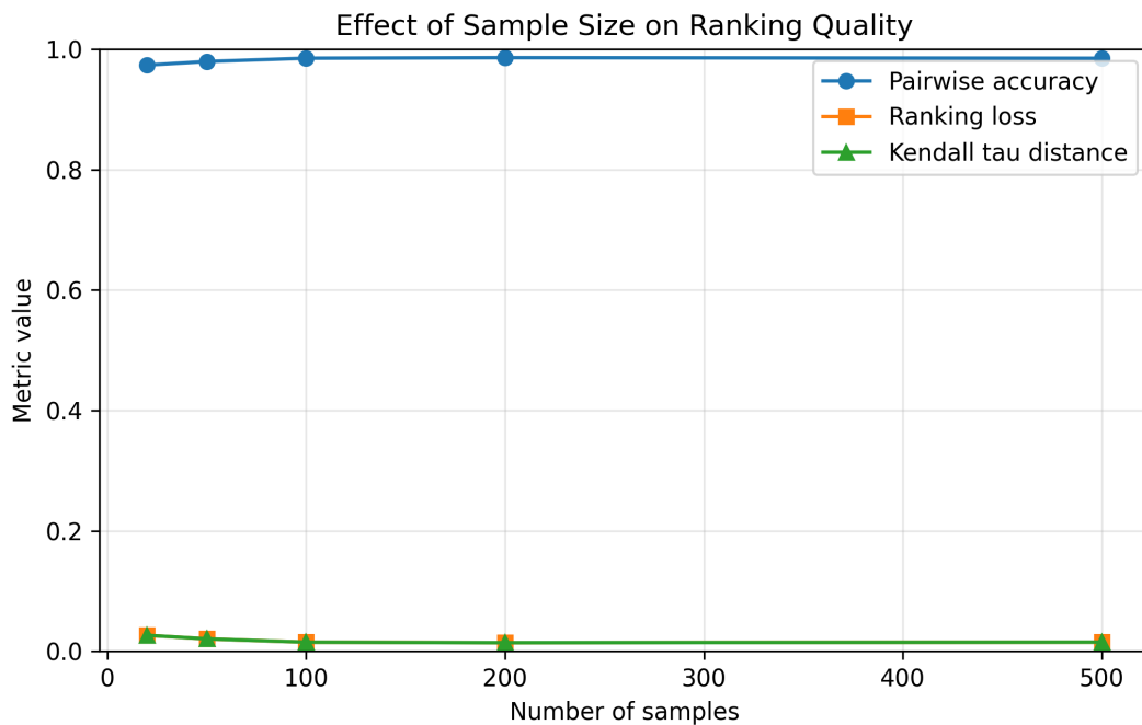
Hình 5: Ảnh hưởng của kích thước mẫu đến chất lượng ranking. Khi số mẫu tăng, pairwise accuracy nhìn chung tăng và ranking loss giảm, sau đó ổn định ở mức tốt.
