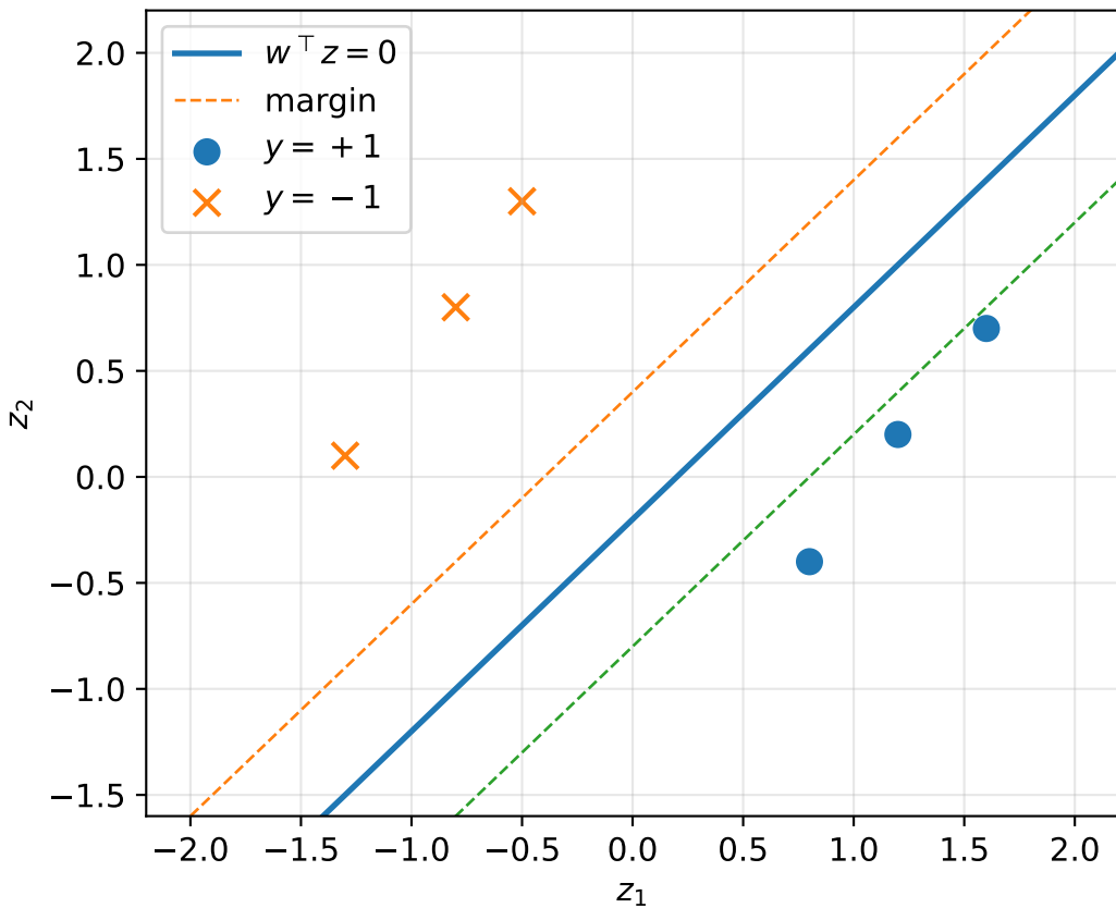
Hình học của SVM-ranking trên vector hiệu z
