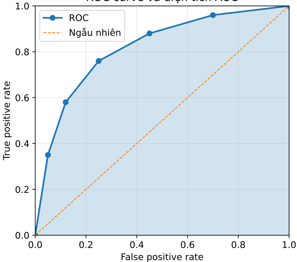
ROC curve và diện tích AUC
