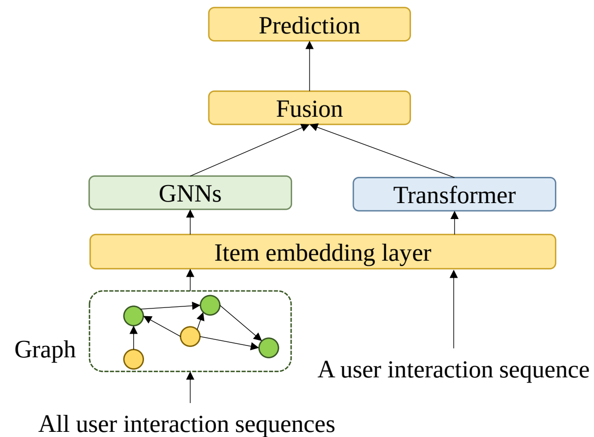
(d) GNNs and Transformer in parallel
