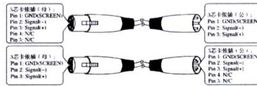
三芯卡侬插 (Canon) DMX512接口线路
