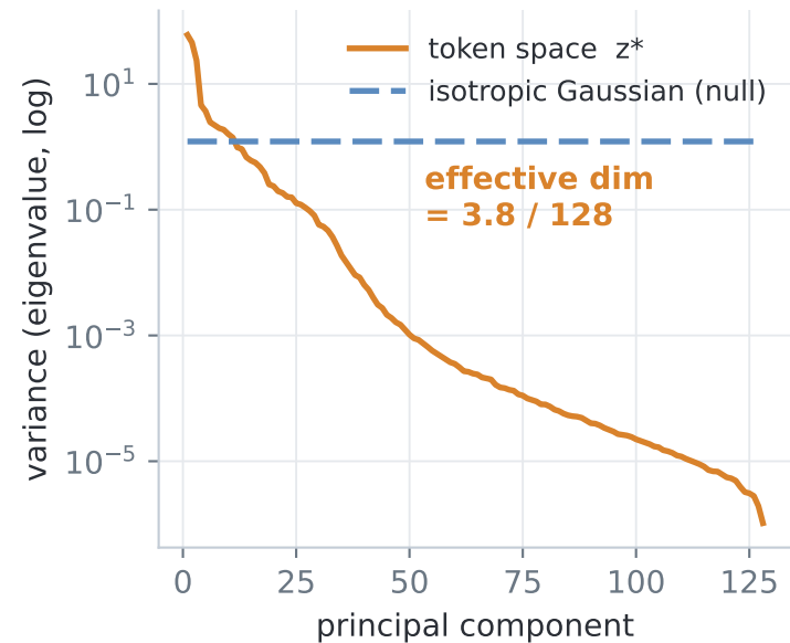
A Eigenvalue spectrum
