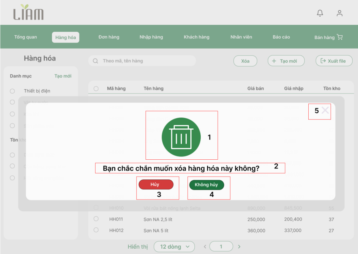
Hình Màn hình Xác nhận xóa hàng hóa
