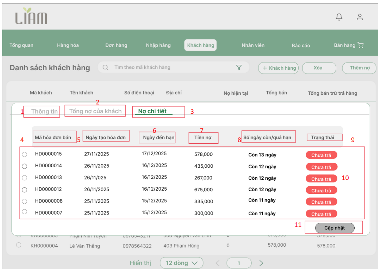
Hình Màn hình xem chi tiết nợ của khách
