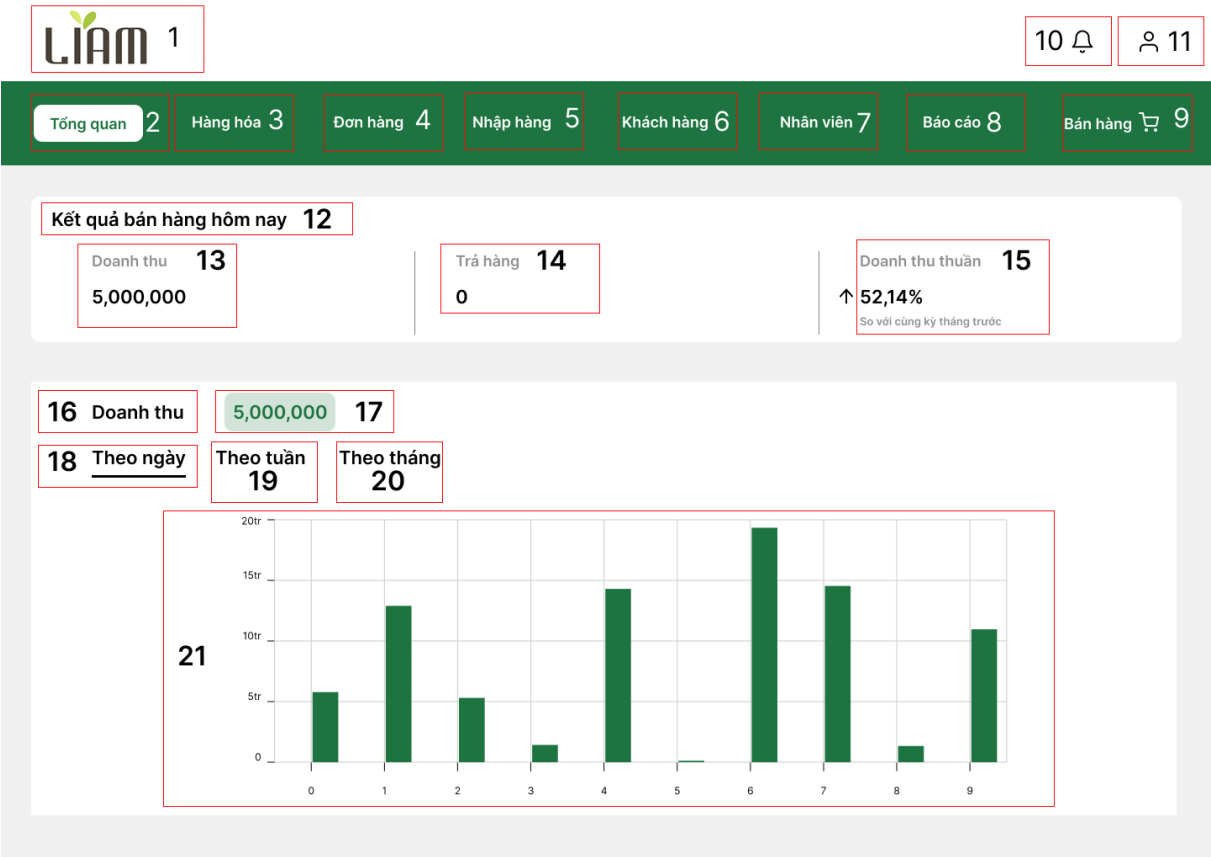
Hình Màn hình Tổng quan
