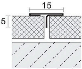
DM-STP145-15W
