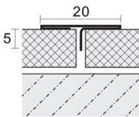
DM-STP145-20W
