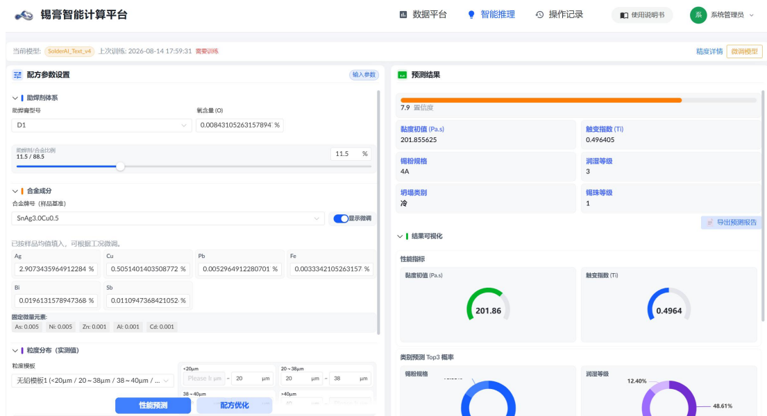
图 15 锡膏性能预测结果页面
