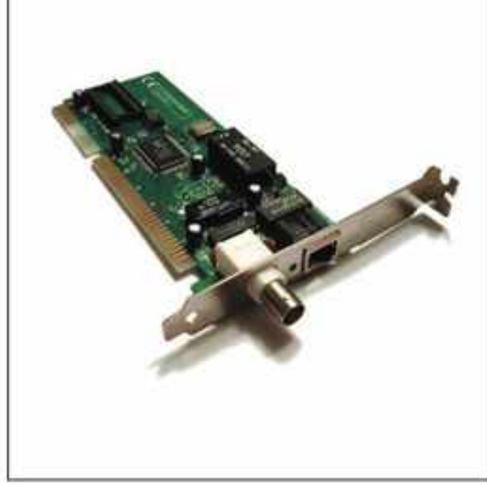
வலையமைப்பு இடைமுக அட்டை (Network Interface Card - NIC)
