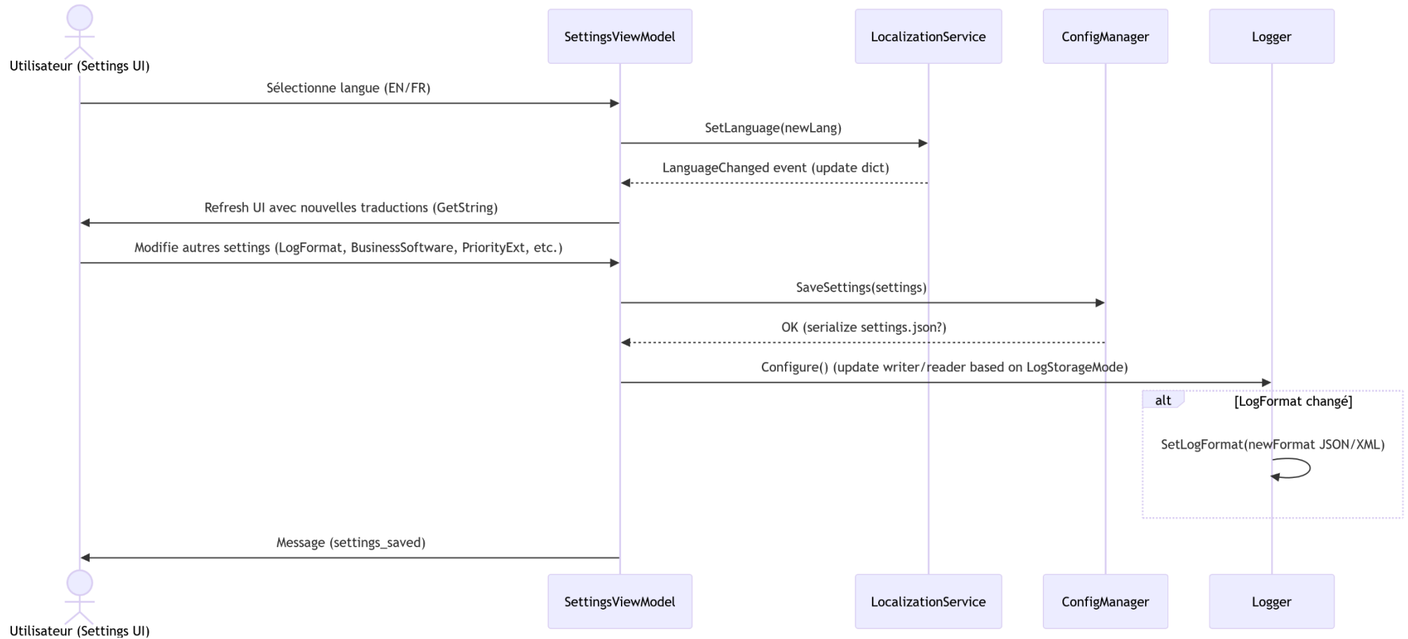
Séquence : Changement de Langue et Sauvegarde Settings
