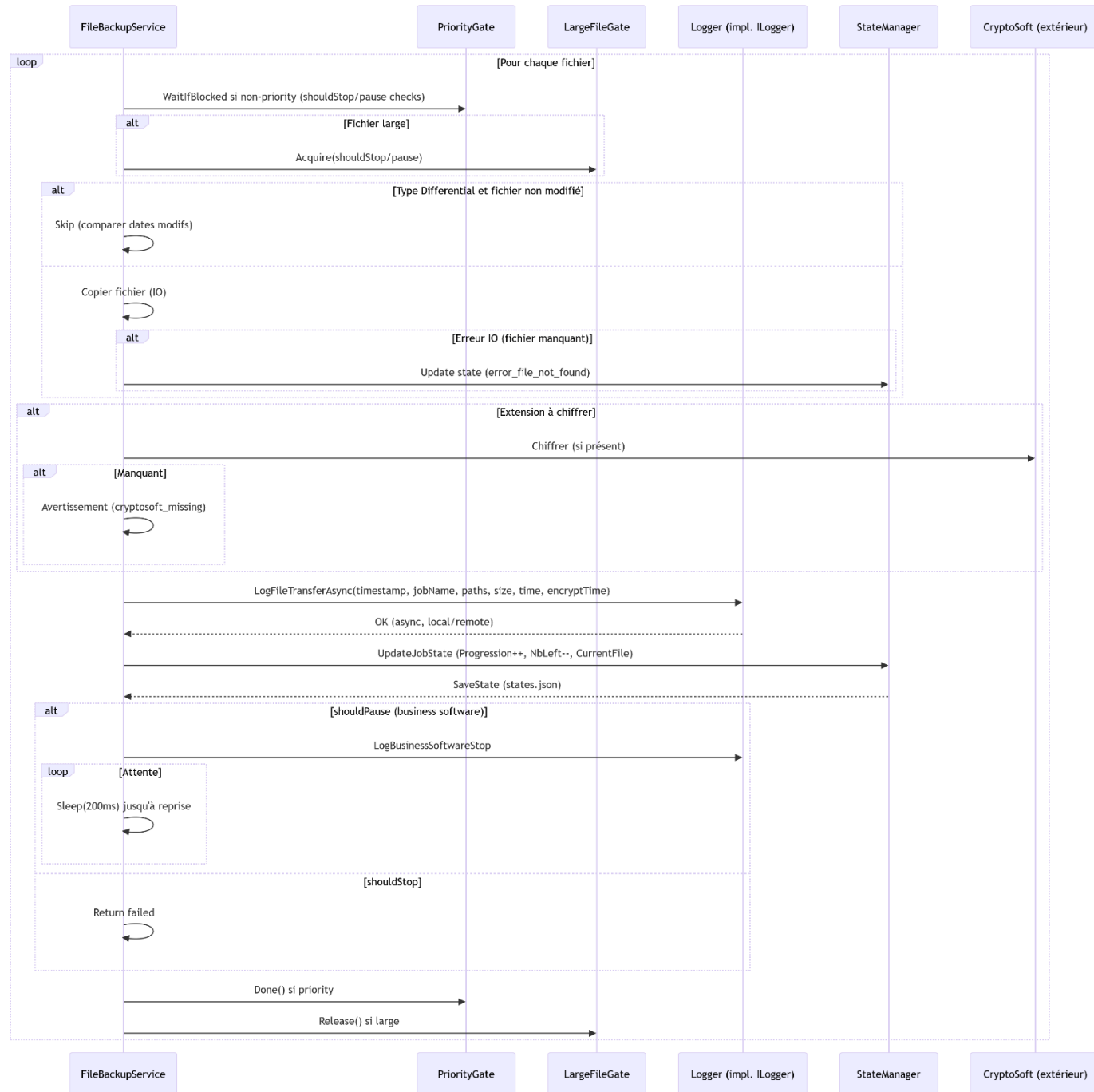
Séquence : Copie Fichiers pendant Backup (Détail sur un Fichier)
