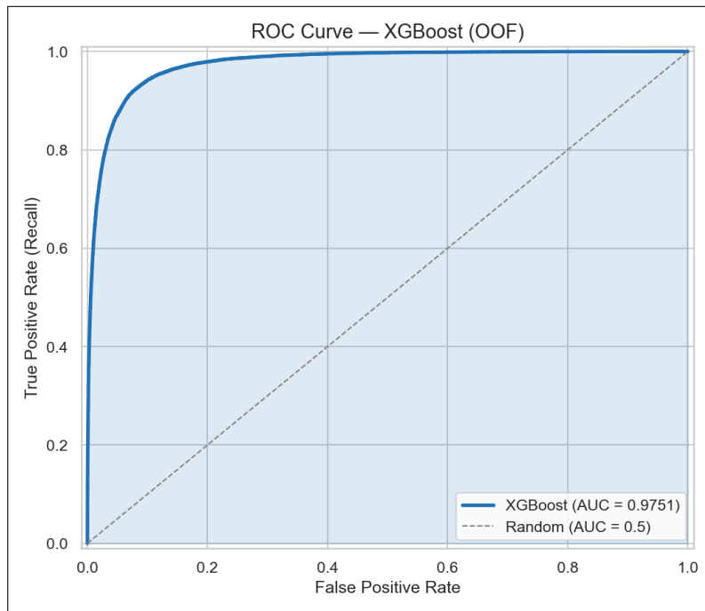
Hình 17: Đường cong ROC — XGBoost (OOF), \text{AUC} = 0,9751
