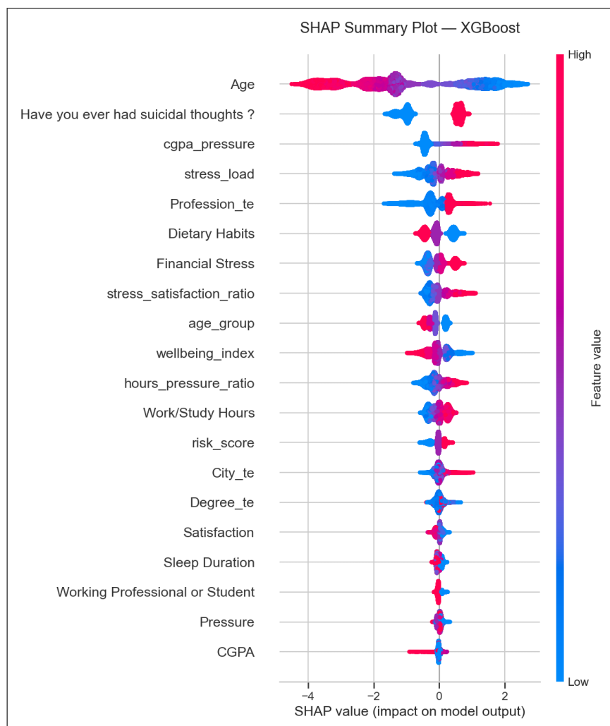
Hình 19: SHAP Summary Plot — XGBoost: mỗi điểm là một mẫu, màu đỏ = giá trị cao, xanh = giá trị thấp
