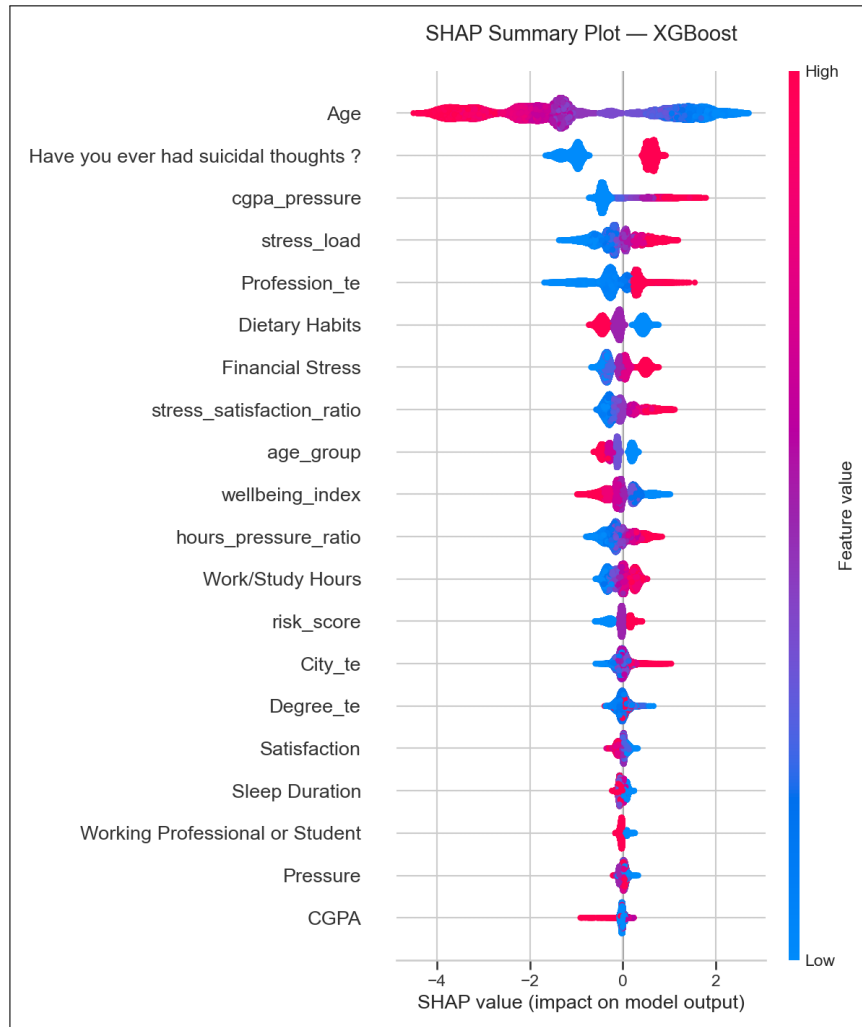
Hình 19: SHAP Summary Plot — XGBoost: mỗi điểm là một mẫu, màu đỏ = giá trị cao, xanh = giá trị thấp
