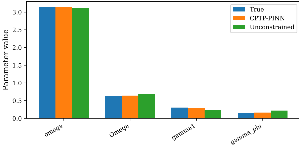
Parameter Recovery
