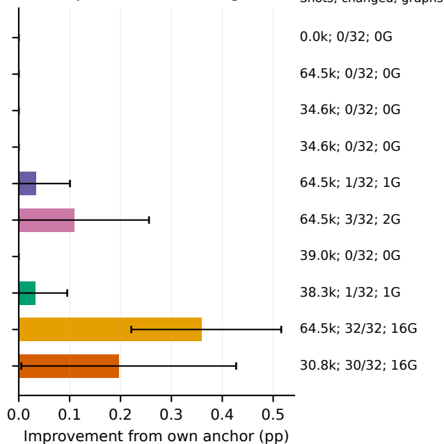
(d) p = 3 : refinement gain
