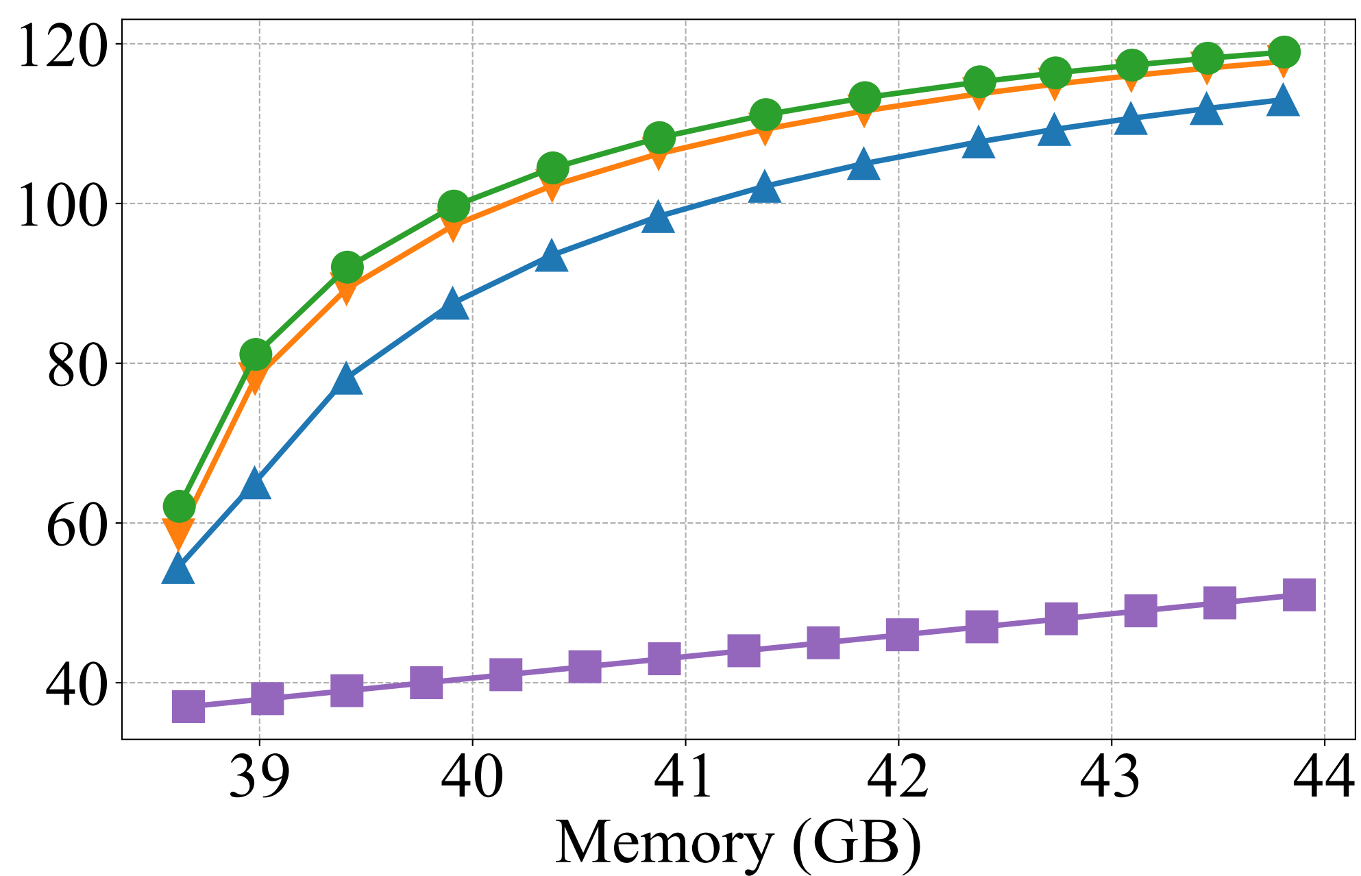
SIFT100M
