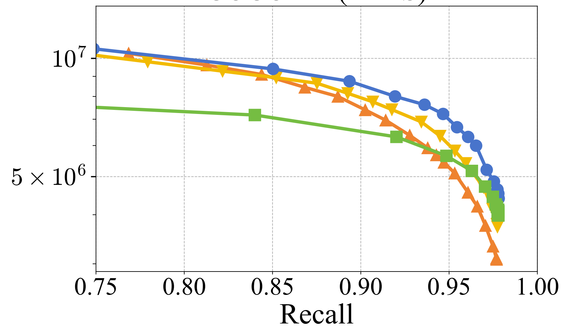
COCO-I2I (PARS)
