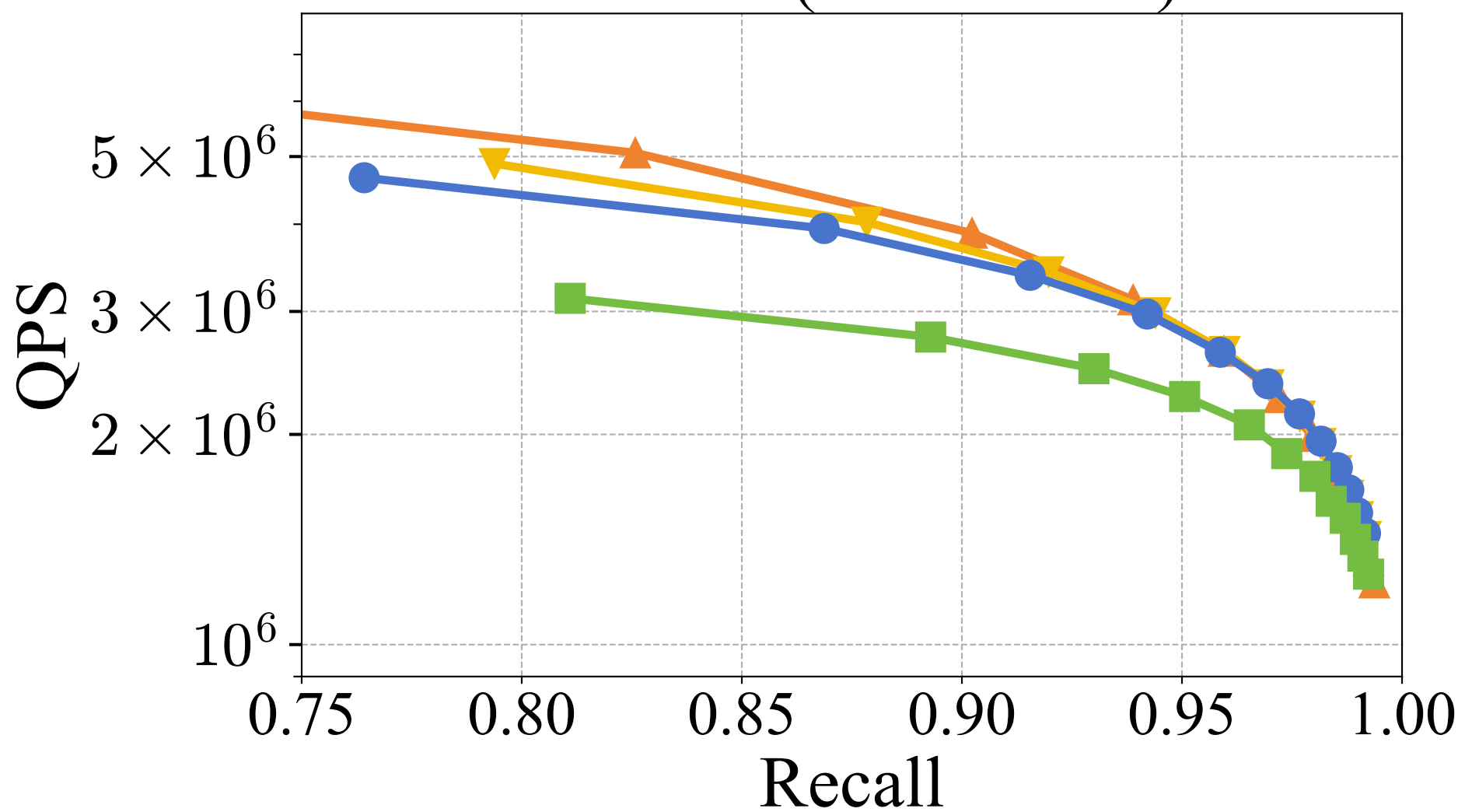
SIFT1M (PARS-Base)
