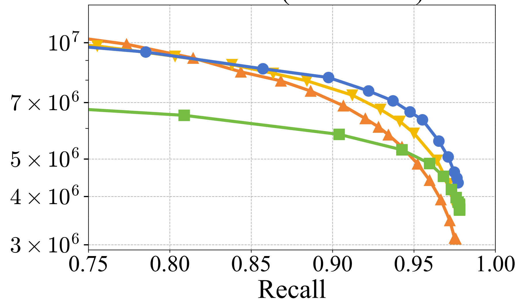
COCO-I2I (PARS-Base)
