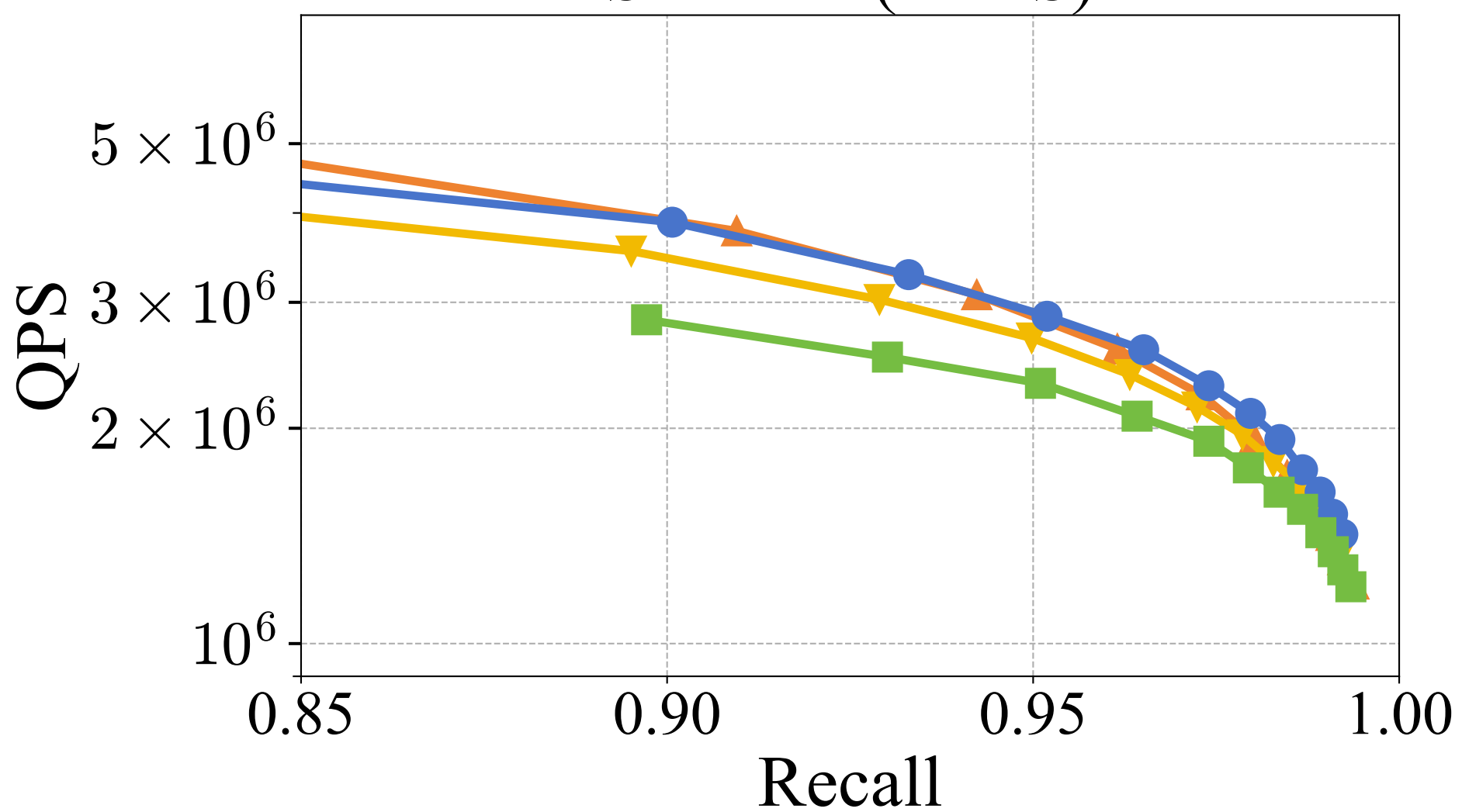
SIFT1M (PARS)
