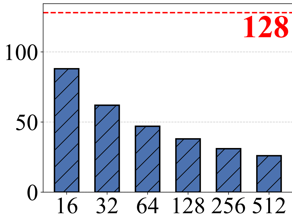
SIFT1M
