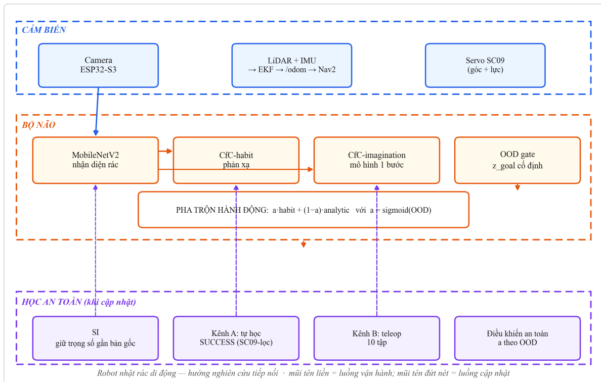
Hình H: Sơ đồ khối hệ thống robot nhặt rác — hướng nghiên cứu tiếp nối. Camera → MobileNetV2 (nhận diện rác) → Cfc-habit (phản xạ) và Cfc-imagination (mô hình 1 bước); LiDAR+IMU → EKF → Nav2 (định vị, di chuyển); Servo SC09 (góc + lực — tín hiệu grasp). OOD gate so với z\_goal sinh \alpha = \text{sigmoid}(\text{OOD}) để trộn hành động với điều khiển giải tích. Mũi tên đứt nét = luồng cập nhật khi học: SI giữ trọng số, Kênh A tự học (SUCCESS qua tín hiệu SC09), Kênh B teleop. Phần cứng: khung chassis, 2 cụm 3S, 2 buck 5V, L298N.
