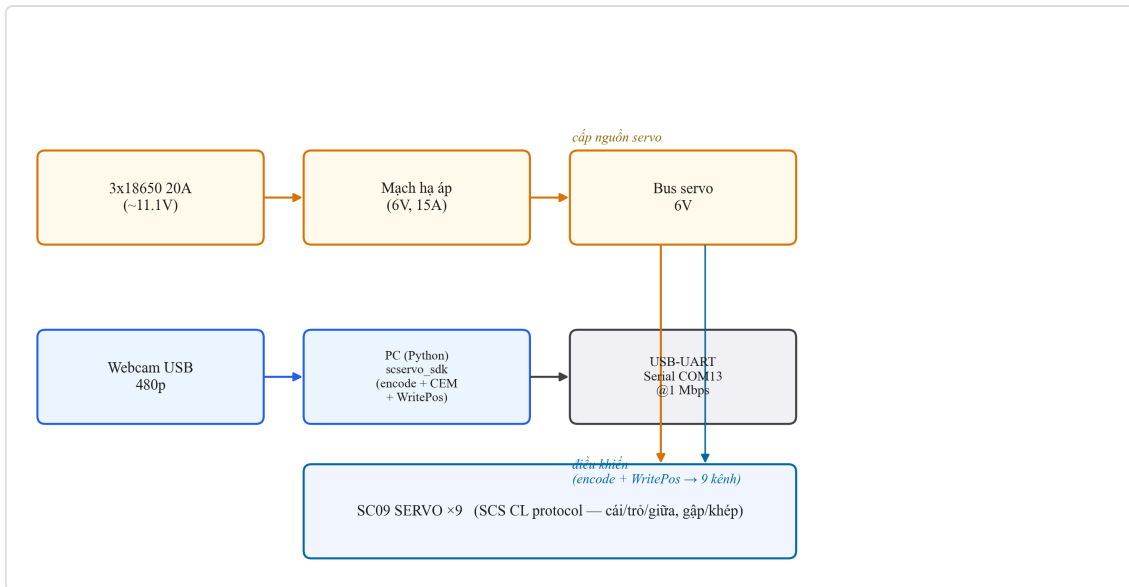
Hình B2: Sơ đồ kết nối phần cứng
