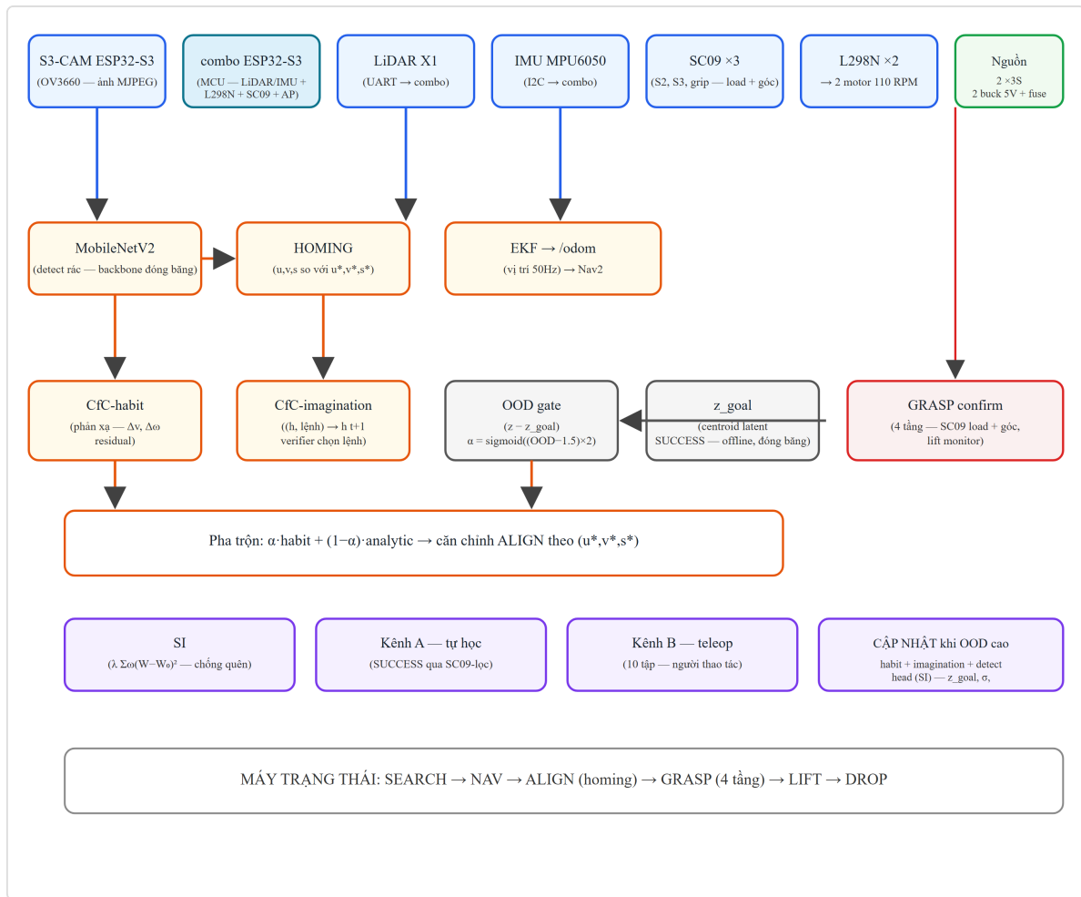
Hình H: Sơ đồ khối hệ thống robot nhặt rác — hướng nghiên cứu tiếp nối. Camera → MobileNetV2 (nhận diện rác) → HOMING ( u^*, v^*, s^* — căn chỉnh điểm grasp); LiDAR+IMU → EKF → Nav2 (định vị, di chuyển). CfC-habit (phản xạ) chống CfC-imagination (mô hình 1 bước — kiểm chứng);
