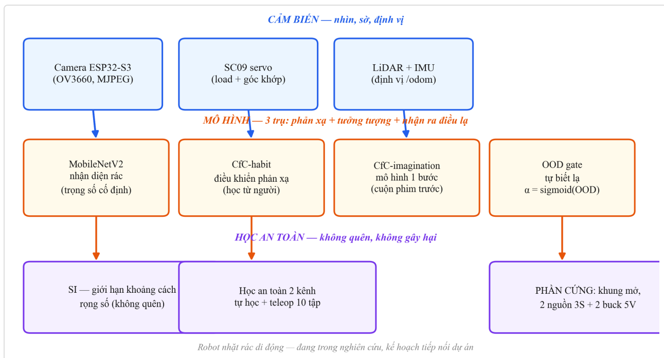
Hình H: Sơ đồ khối hệ thống robot nhặt rác di động — hướng nghiên cứu tiếp nối
