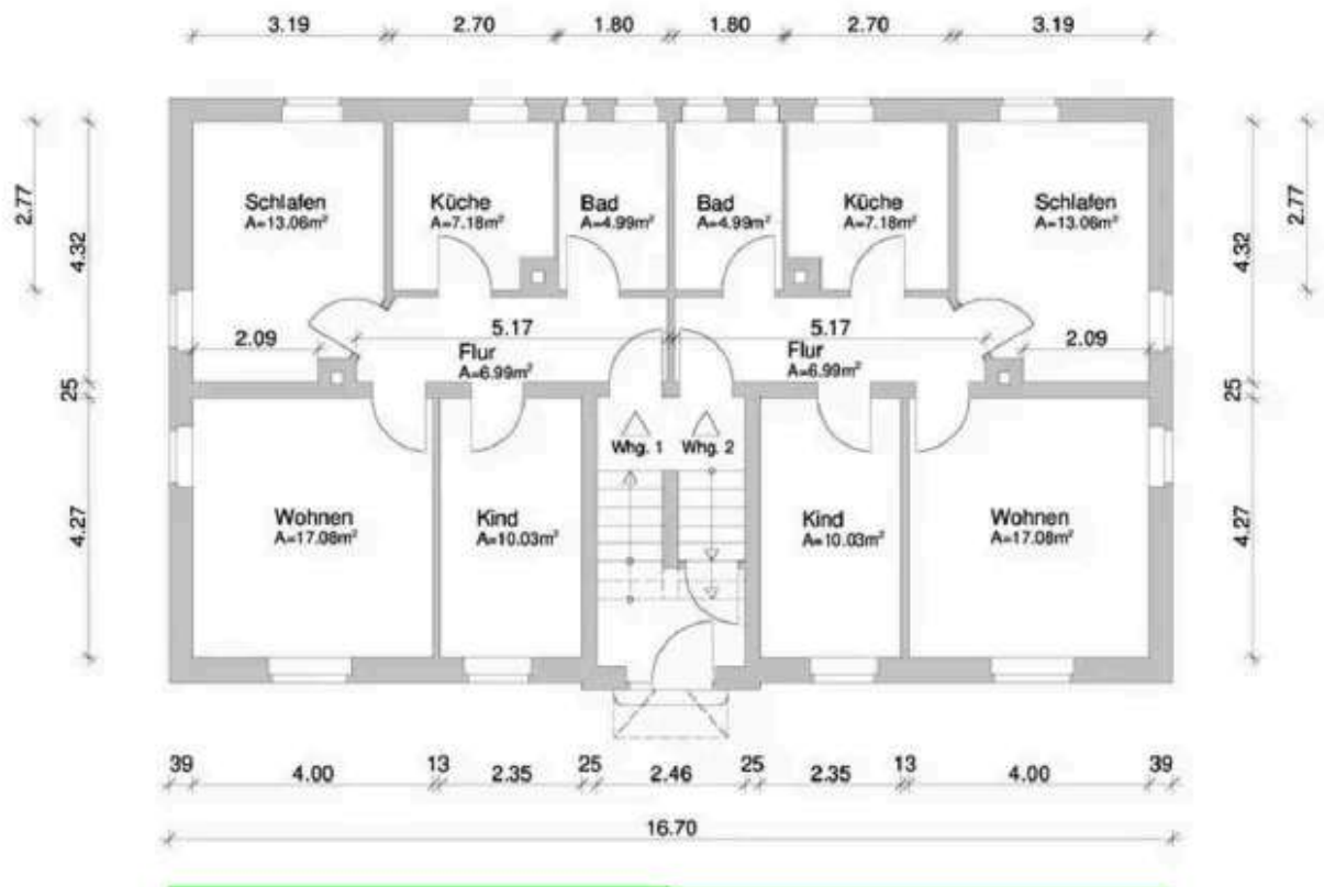
Grundriss Erdgeschoss
