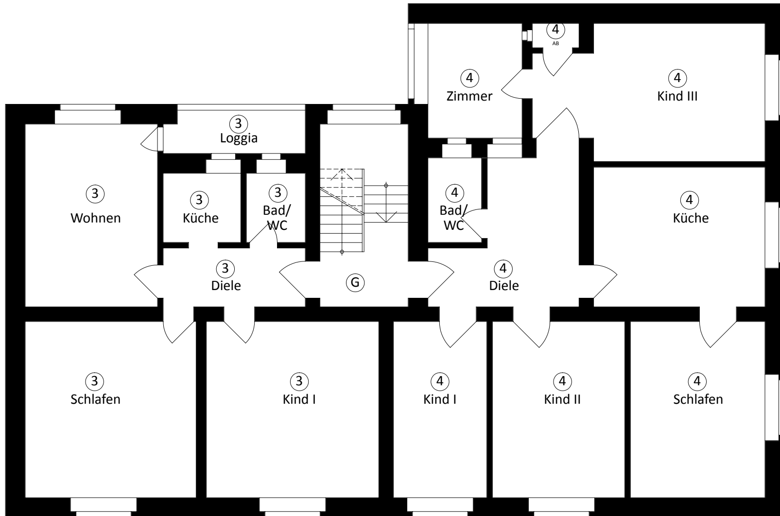
1. Obergeschoss 1:100
