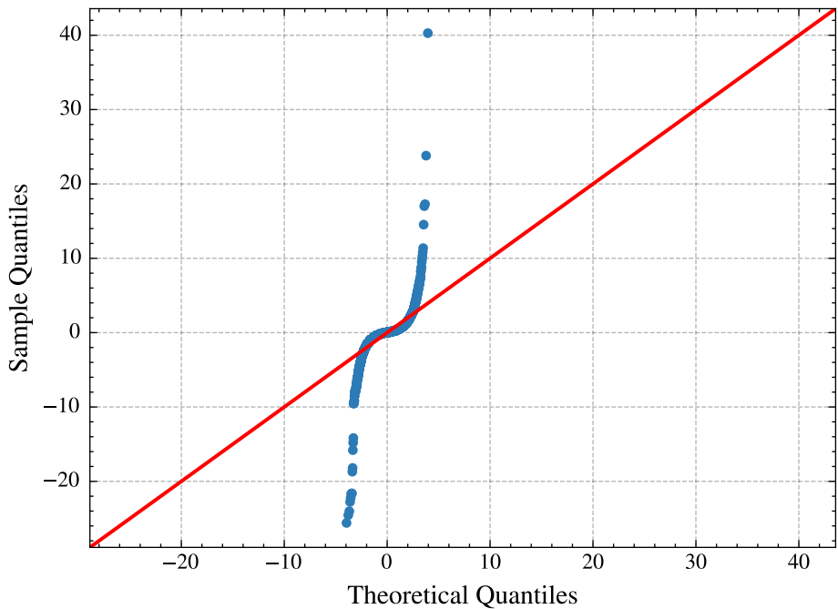
Q-Q Plot — Iso_width
