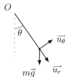
(3) pendule
