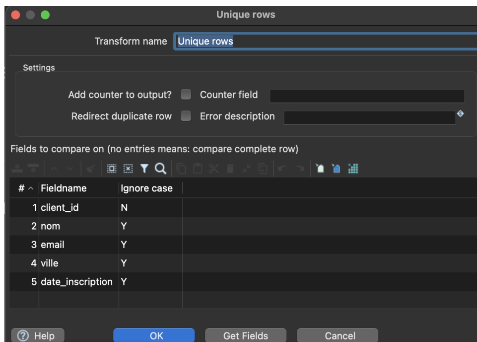
FIGURE 22 – Configuration de la déduplication des clients.
