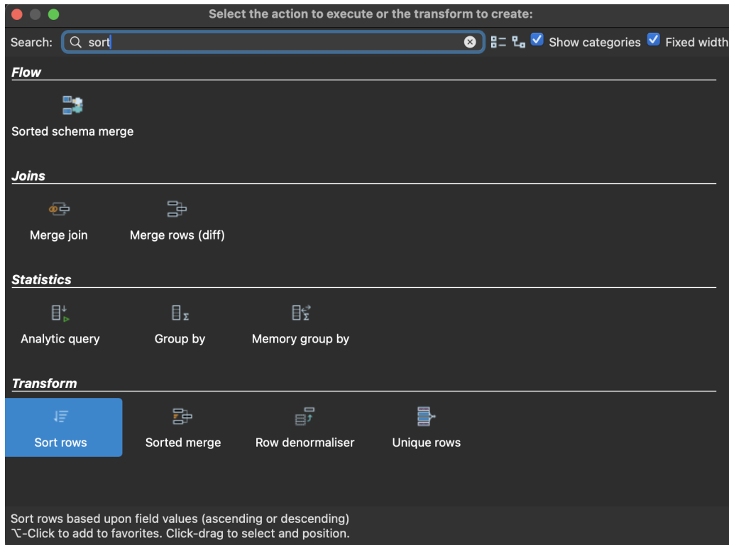
FIGURE 19 – Ajout de la transformation Sort rows .
