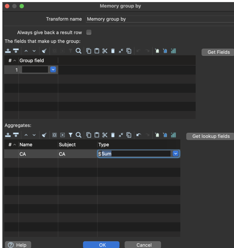
FIGURE 30 – Paramétrage d'une première agrégation : somme du champ CA .
