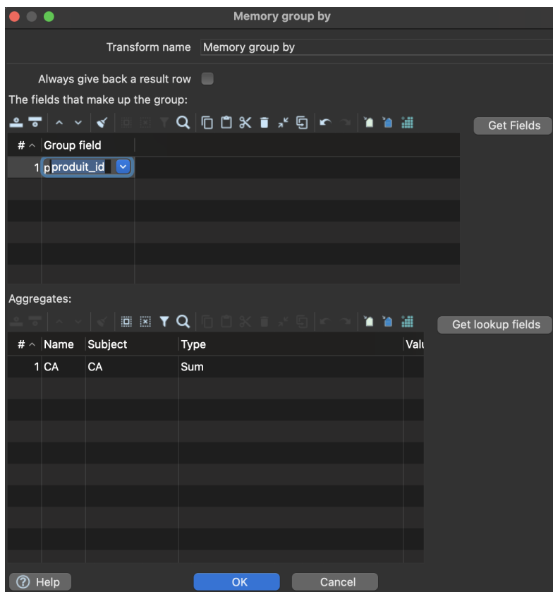
FIGURE 33 – Agrégation du CA par produit (regroupement sur produit_id ).
