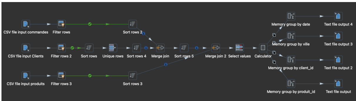
FIGURE 1 – Vue d'ensemble : le pipeline ETL complet construit dans ce tutoriel.
