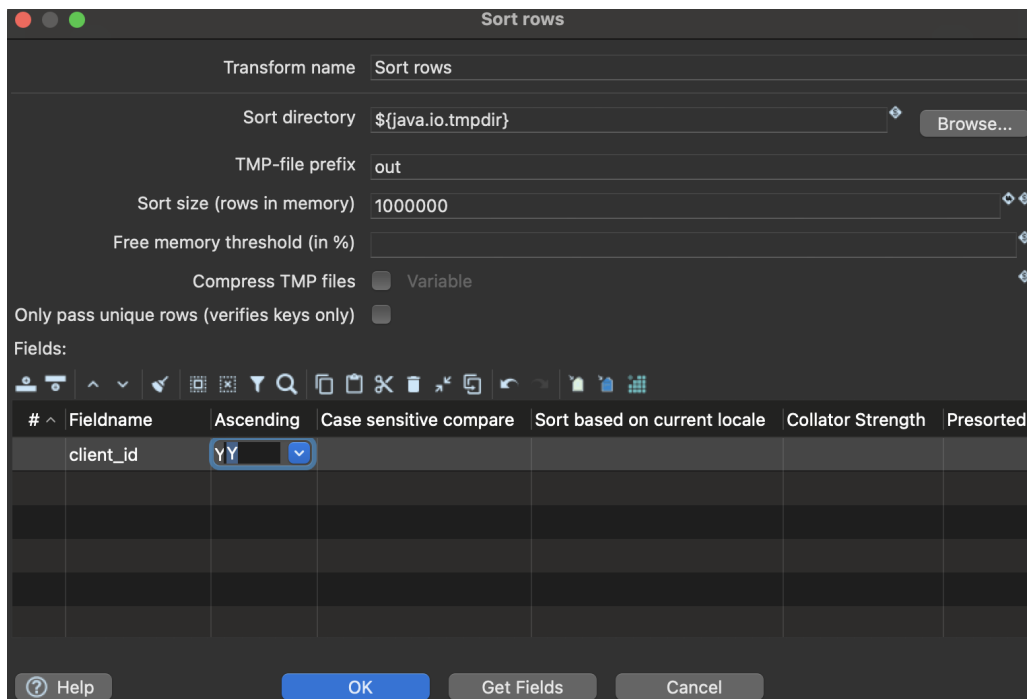
FIGURE 20 – Tri sur la clé client_id .
