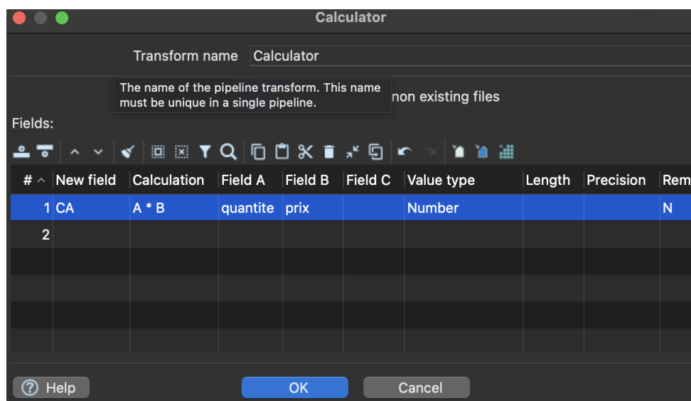
FIGURE 28 – Définition du champ CA = \text{quantite} \times \text{prix} .
