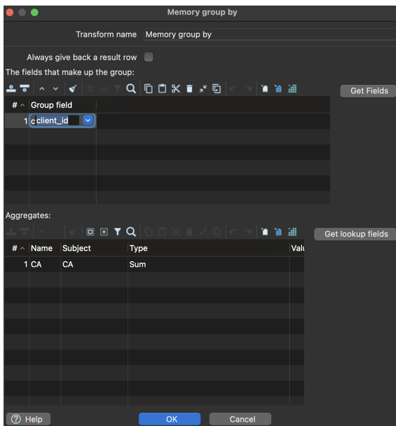
FIGURE 32 – Agrégation du CA par client (regroupement sur client_id ).
