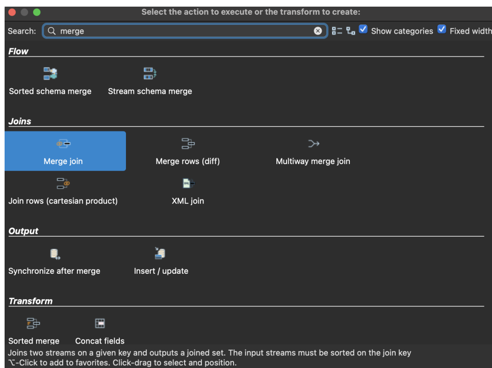
FIGURE 23 – Ajout de la première transformation Merge join .
