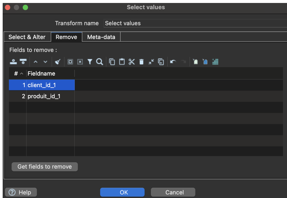
FIGURE 26 – Suppression des champs en double (onglet Remove ).
