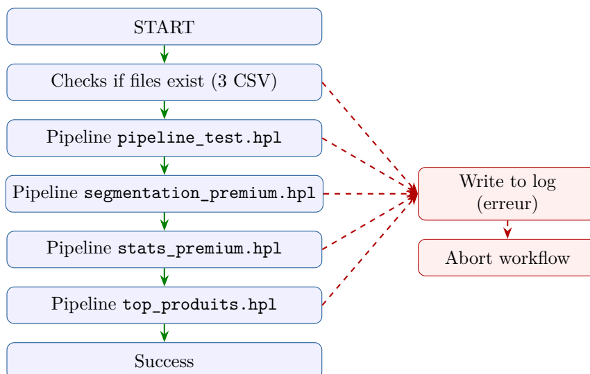
FIGURE 39 – Workflow étendu : enchaînement nominal (flèches pleines) et branche d'échec (pointillés).
