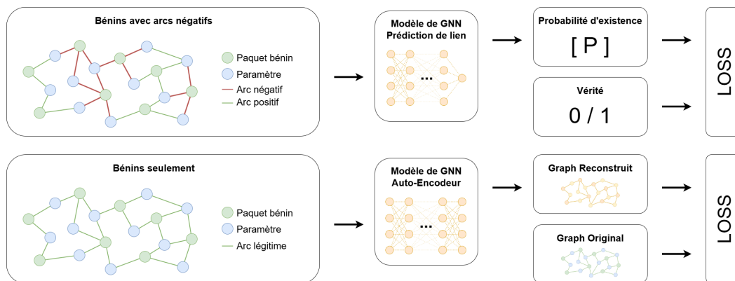
Figure 1.9: Représentation du processus d'apprentissage non supervisé. La première ligne correspond à une tâche de prédiction de lien avec des arcs négatifs artificiels, tandis que la seconde ligne correspond à une tâche de reconstruction.
