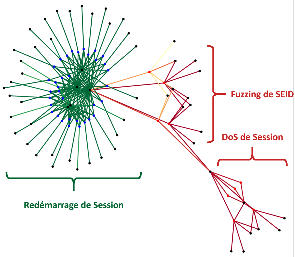
Figure 1.13: Représentation de la prédiction d'anomalie sur un graph représentant un ensemble de paquets observés. Les arcs rouges signalent des anomalies très probables tandis que les arcs verts signalent une faible probabilité d'anomalie. Les paquets bénins sont représentés comme des nœuds de couleur bleu et les paquets d'attaques comme des nœuds de couleur rouge.
