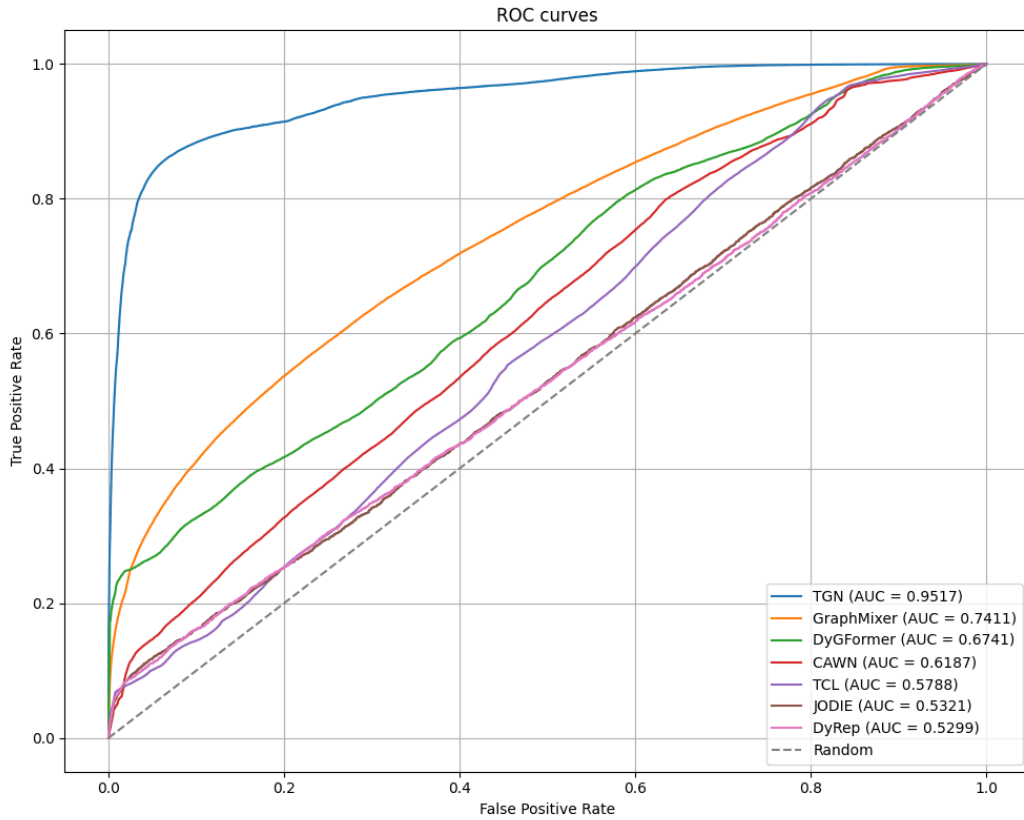
Figure 1.8: Courbes ROC pour les différents modèles de prédiction de lien supervisés.
