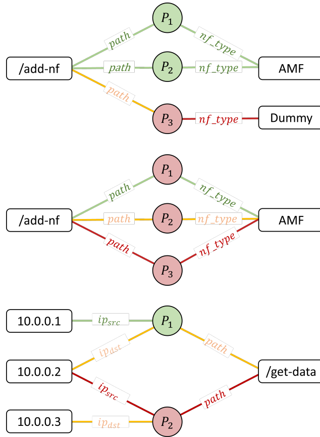
Figure 1.12: Représentation des coefficients d'anomalies pour les dimensions (a) sémantique, (b) séquentielle, et (c) topologique. Les nœuds rouges représentent des paquets d'attaque tandis que les verts représentent des paquets bénins.
