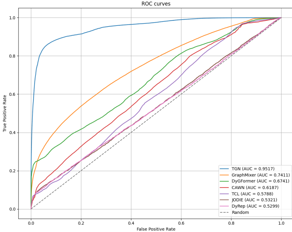
FIGURE 4.8 – Courbes ROC pour les différents modèles de prédiction de lien supervisés.
