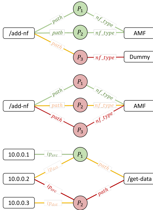
FIGURE 4.12 – Représentation des coefficients d'anomalies pour les dimensions (a) sémantique, (b) séquentielle, et (c) topologique. Les nœuds rouges représentent des paquets d'attaque tandis que les verts représentent des paquets bénins.
