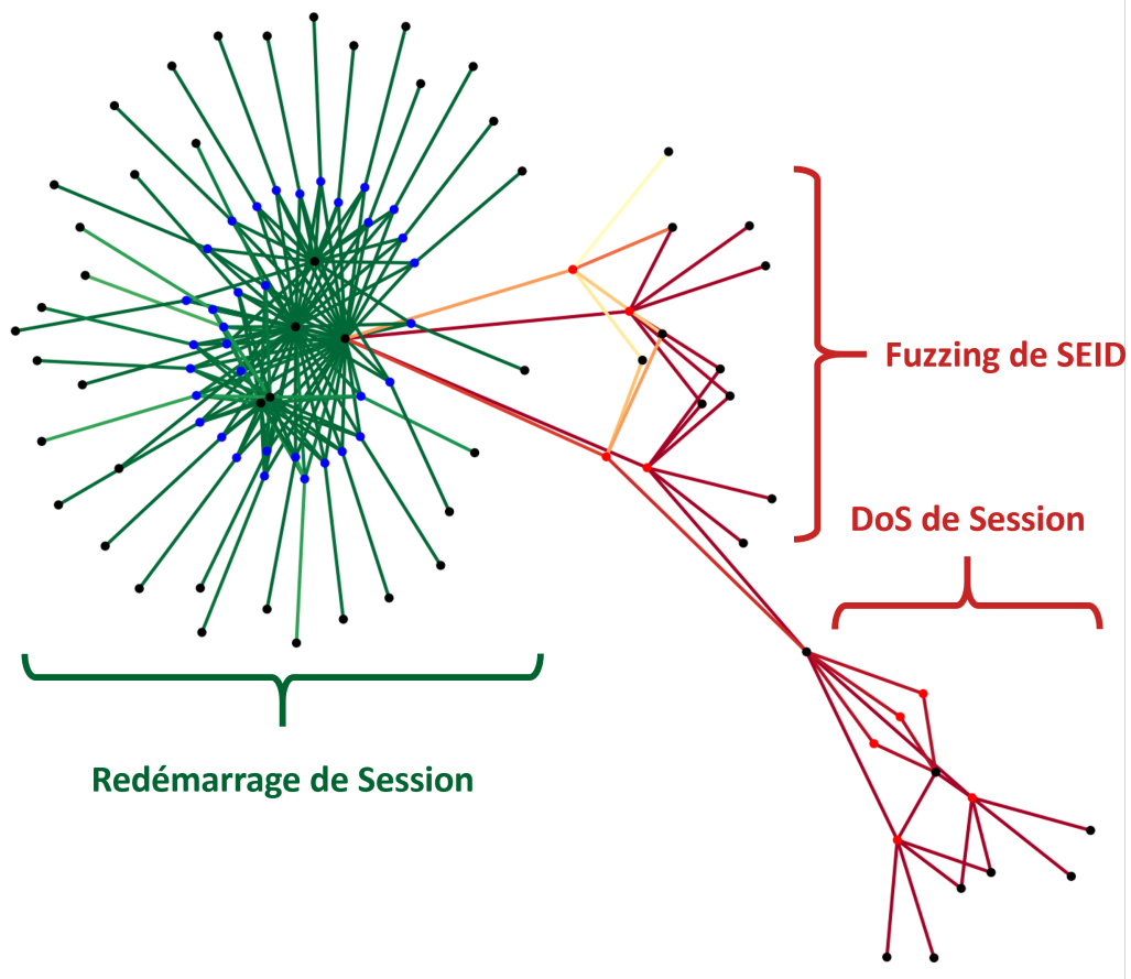
FIGURE 4.13 – Représentation de la prédiction d’anomalie sur un graph représentant un ensemble de paquets observés. Les arcs rouges signalent des anomalies très probables tandis que les arcs verts signalent une faible probabilité d’anomalie. Les paquets bénins sont représentés comme des nœuds de couleur bleu et les paquets d’attaques comme des nœuds de couleur rouge.
