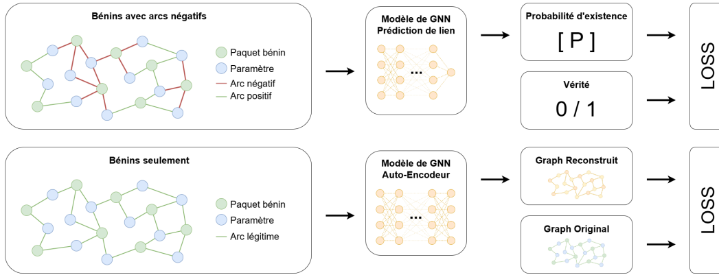
FIGURE 4.9 – Représentation du processus d’apprentissage non supervisé. La première ligne correspond à une tâche de prédiction de lien avec des arcs négatifs artificiels, tandis que la seconde ligne correspond à une tâche de reconstruction.
