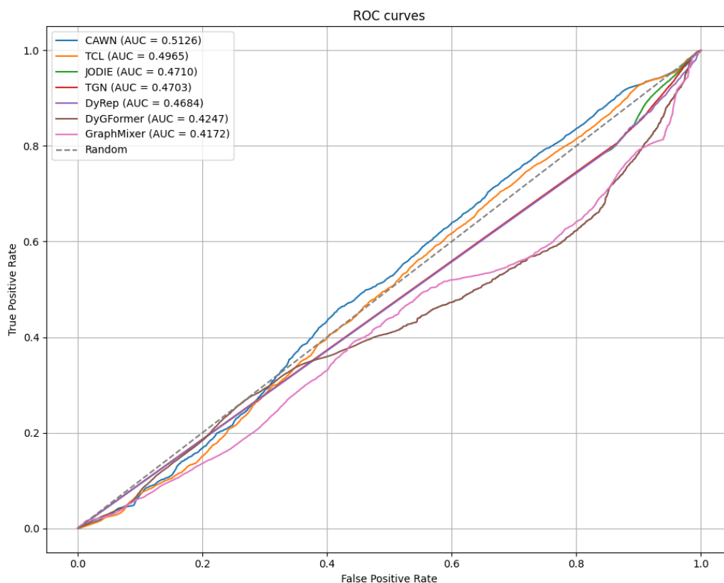
FIGURE 4.10 – Courbes ROC pour les différents modèles de prédiction de lien non supervisés.
