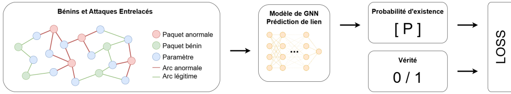
Figure 1.6: Représentation du processus d'apprentissage supervisé.
